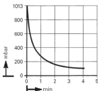
Tempo di svuotamento di un recipiente da 20 l
